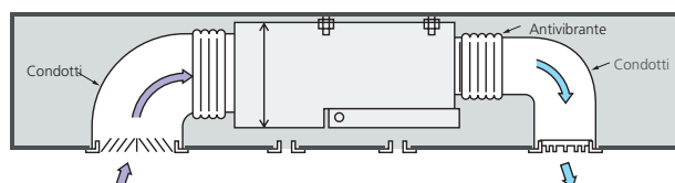
Unità interna ultra-sottile
